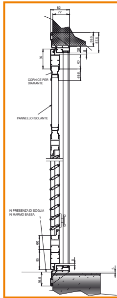
Telaio serie PLUS su 4 lati
